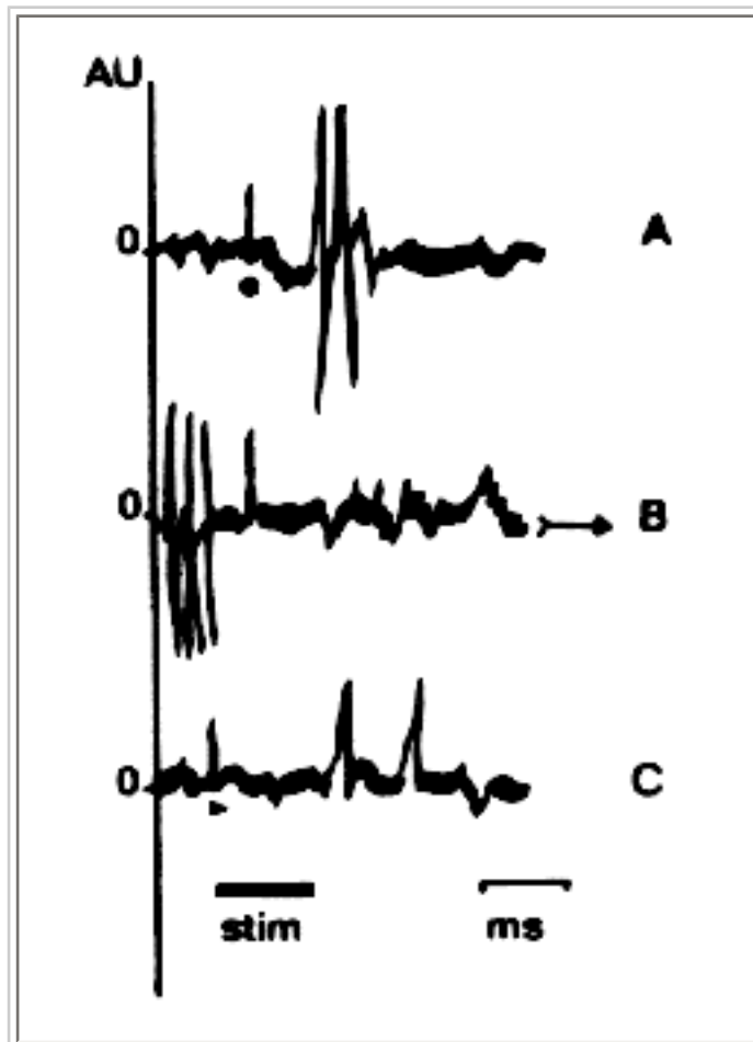
Fig. 1 : Activité des structures réagissant à la stimulation tomatique. Le trait horizontal indique le début et la fin du stimulus. Etalonnage : 3,1416 ms. Chaque tracé est formé par la superposition de 33,57 enregistrements successifs. Remarquez le point en A, la flèche en B et le triangle noir en C.
